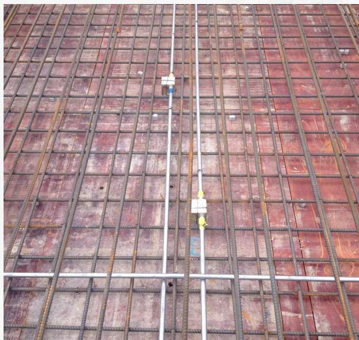
镀锌管管暗敷横平竖直，间距一致，绑扎牢固线盒及外露管成品保护到位
