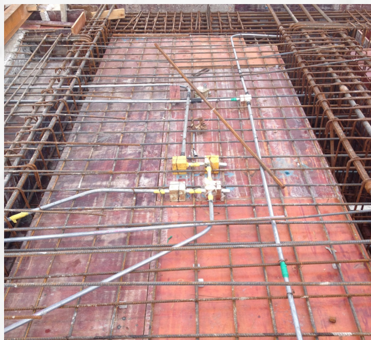
镀锌管管暗敷横平竖直，间距一致，绑扎牢固线盒及外露管成品保护到位
