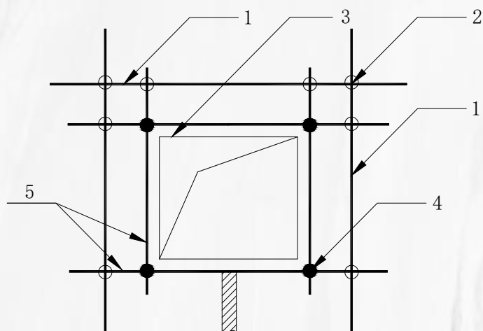
1-主筋 2-12#铅丝绑扎 3-线盒 4-电焊 5-附加钢筋
